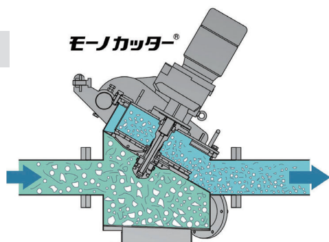
「日本下水道事業団 機械設備標準仕様書」 第10章 第5節 §2 一軸汚泥細断機（インライン型）に適合
