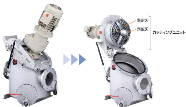
「日本下水道事業団 機械設備標準仕様書」 第10章 第5節 §2 一軸汚泥細断機（インライン型）に適合
